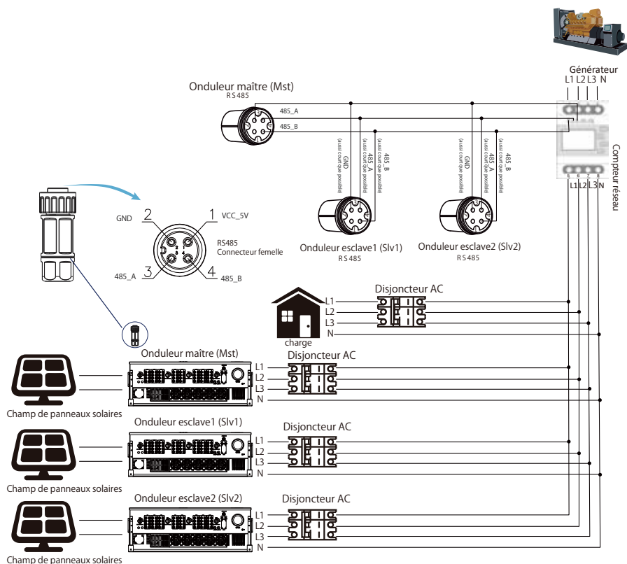
Image 7.23 Schéma de connexion Eastron (table de passage)
