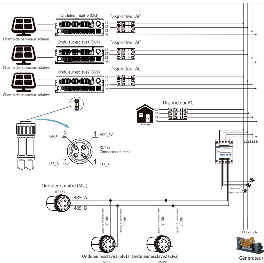
Image 7.35 Schéma de connexion CHINT (table de passage)
