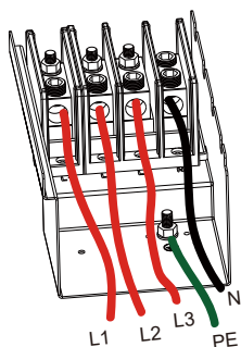
Image 5.9 Connexion des câbles AC aux bornes
