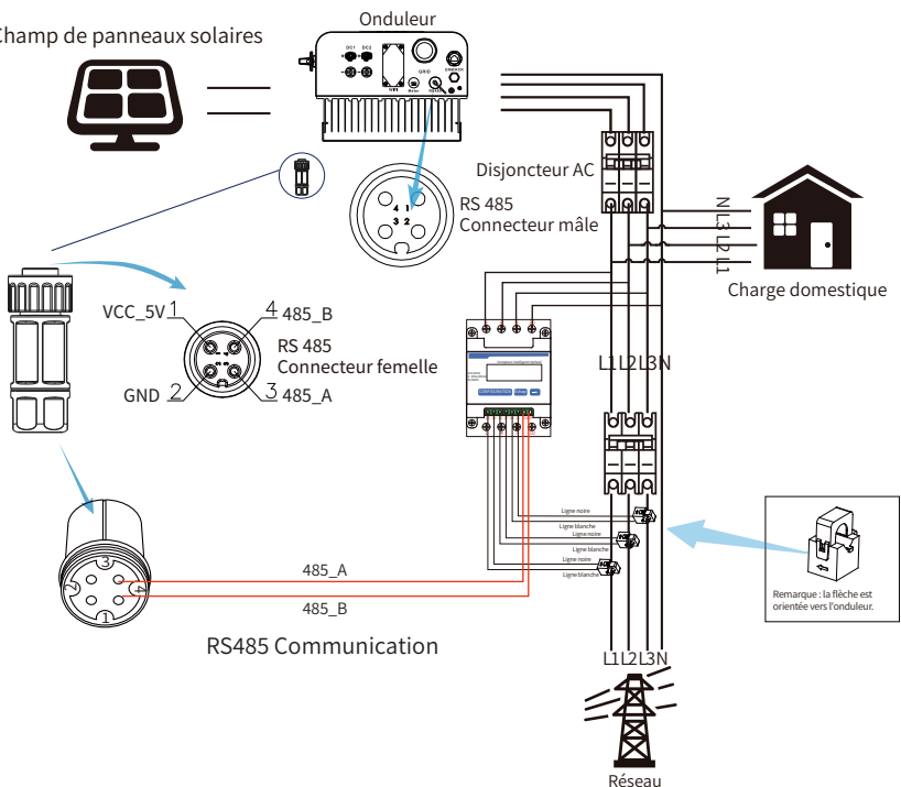
Image 7.14 Schéma de connexion du compteur CHINT
