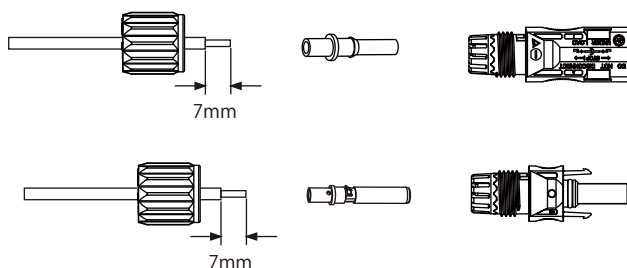
Image 5.3 Démontage de l'écrou de capuchon du connecteur
