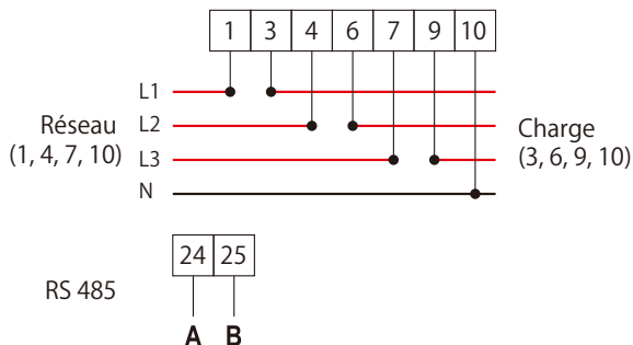
Image 7.28 Compteur CHINT
