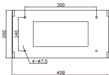
Image 4.5 Installation de la plaque de suspension de l'onduleur
