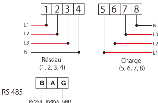
Image 7.3 Compteur Eastron
