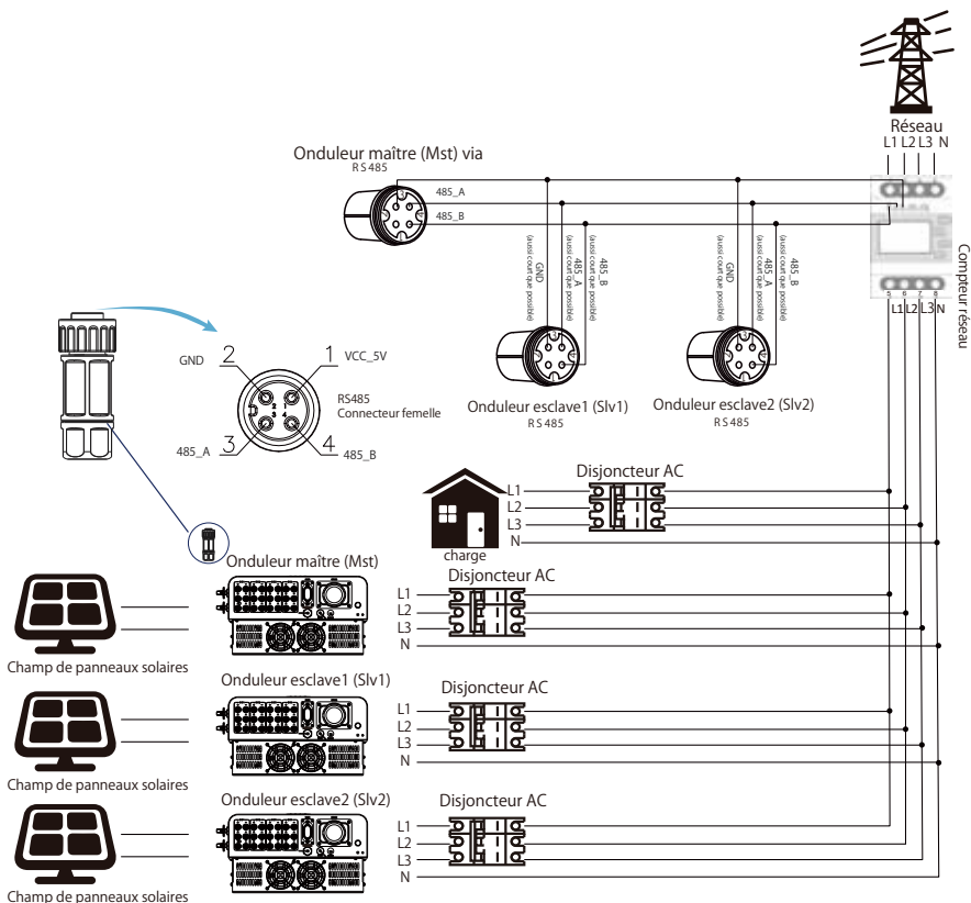
Image 7.19 Schéma de connexion Easton (table de passage)
