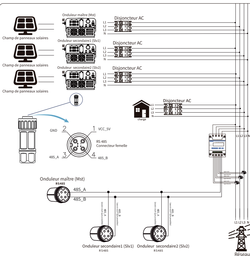
Figure 7.31 Schéma de connexion CHINT (table de passage)
