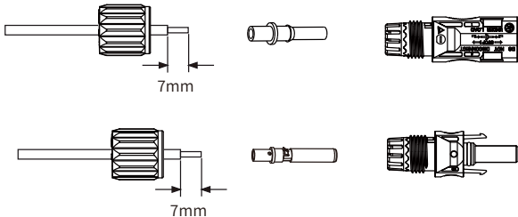
Image 5.3 Démontage de l'écrou de capuchon du connecteur
