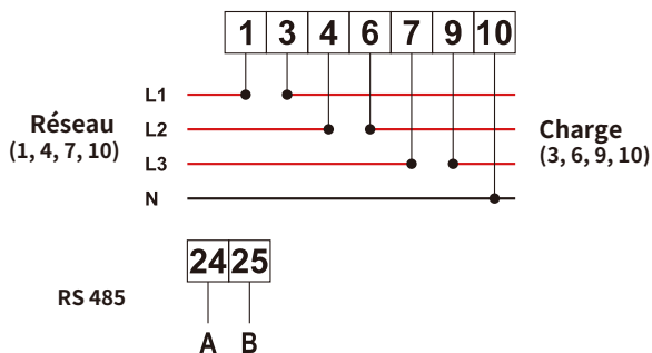
Image 7.9 Compteur CHINT
