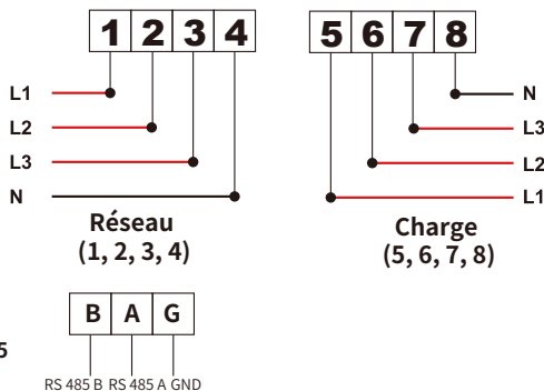
Image 7.1 Compteur Eastron
