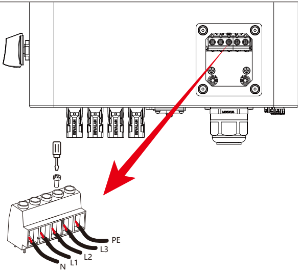
Image 5.7 Connexion d'entrée AC
