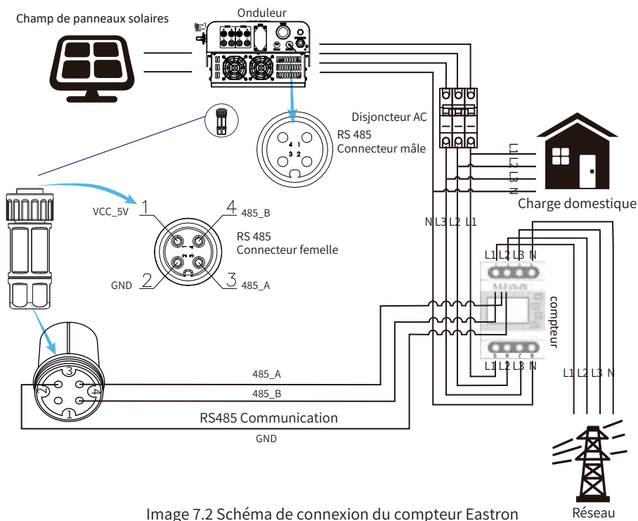
Image 7.2 Schéma de connexion du compteur Eastron
