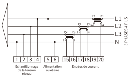
Image 7.24 Compteur Easton
