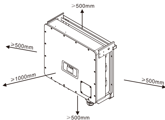
Image 4.3 Espacement entre les onduleurs
