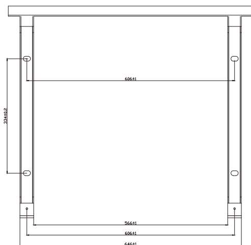
Image 4.4 Dimensions du support de fixation
