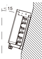
Image 4.2 Angle d'installation
