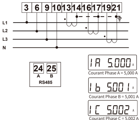
Image 7.32 Compteur CHINT
