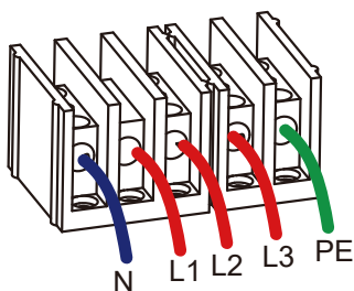
Image 5.9 Connexion des câbles AC aux bornes
