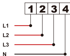
Réseau (1, 2, 3, 4)
