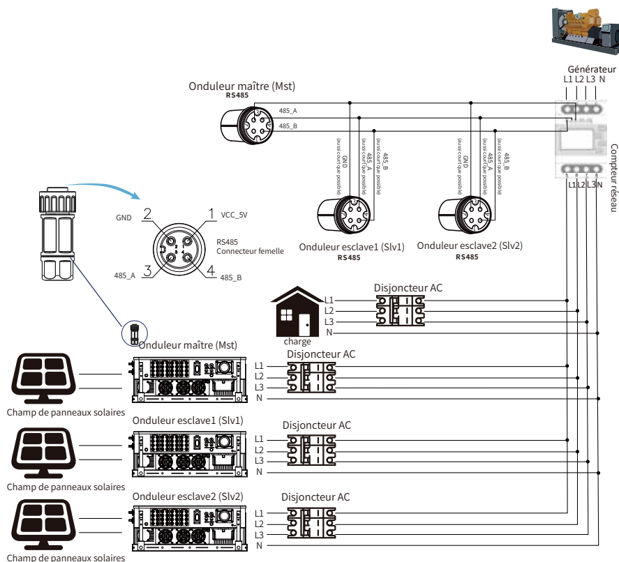
Image 7.23 Schéma de connexion Eastron (table de passage)
