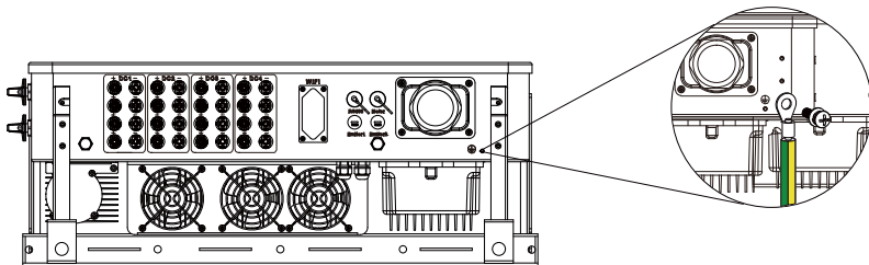
Image 5.11 Installation du conducteur de terre du boîtier
