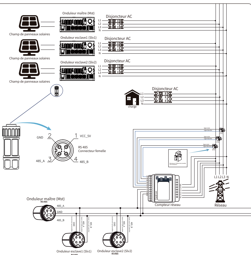
Image 7.25 Schéma de câblage (électricité triphasée)
