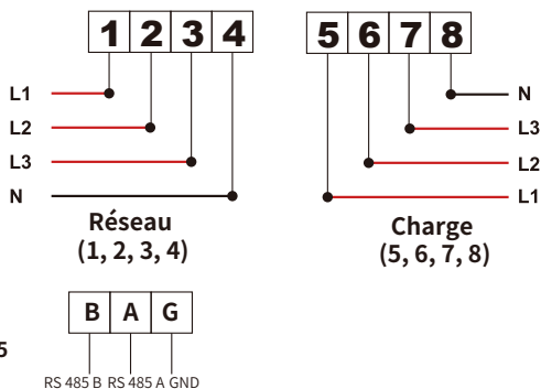
Image 7.3 Compteur Eastron
