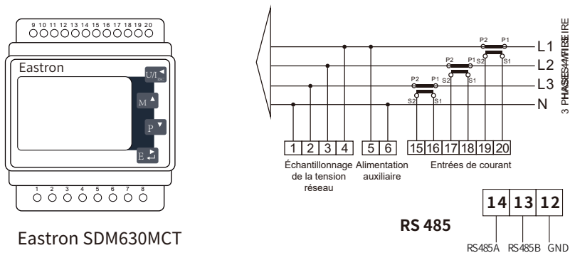
Image 7.24 Compteur Eastron
