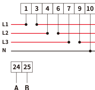
Image 7.11 Compteur CHINT
