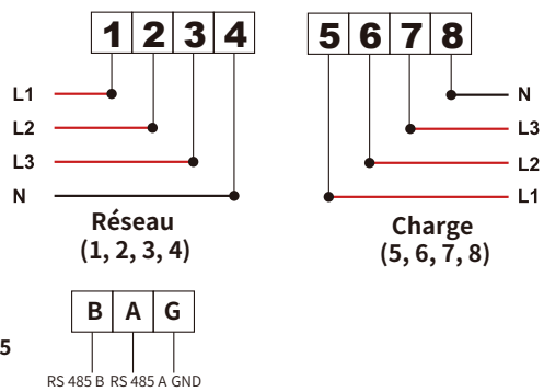
Image 7.3 Compteur Eastron
