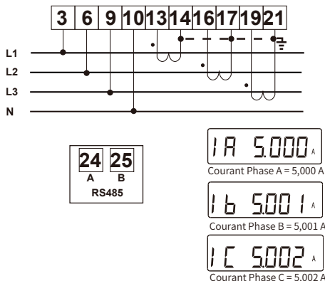
Image 7.32 Compteur CHINT
