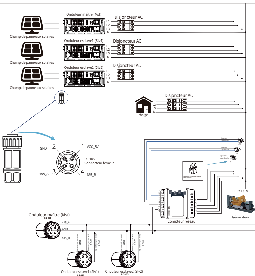
Image 7.26 Compteur Eastron
