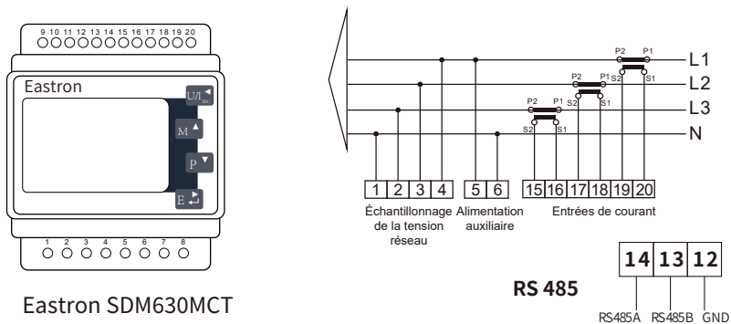
Image 7.26 Compteur Eastron
