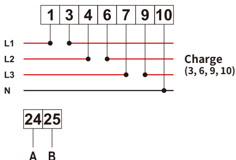
Image 7.9 Compteur CHINT
